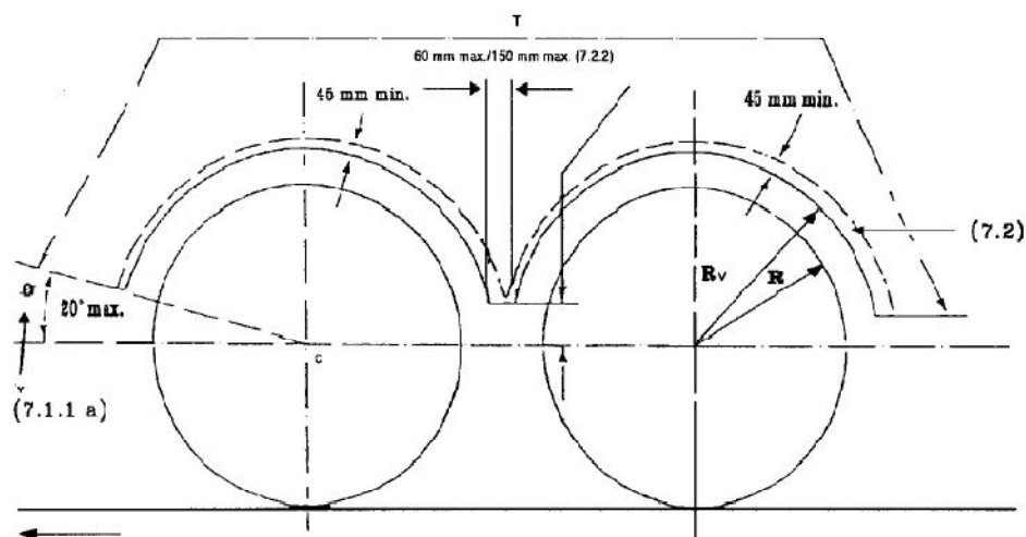
شکل ث: موقعیت نصب گلگیر و باران گیر
