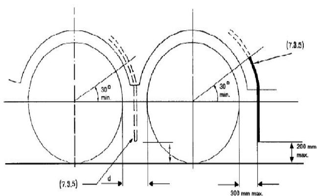
شکل چ: موقعیت تجهیزات ممانعت از پاشش برای محورهای چندتایی
